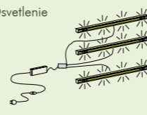
LED - Osvetlenie Typ 125 H Osvetlenie sklenených polic 3 x svetlo, 1 x Trafo 60 W 1 x predlžovací kábel s vypínačom
